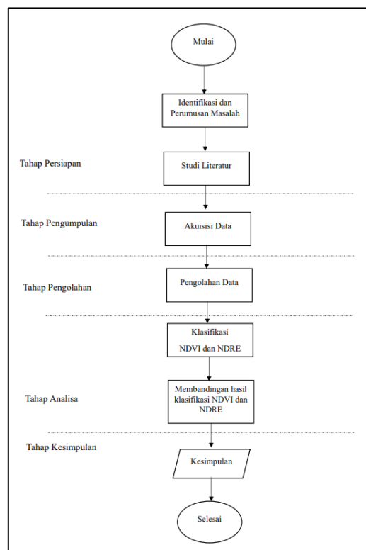
Gambar 1. Kerangka Pemikiran
