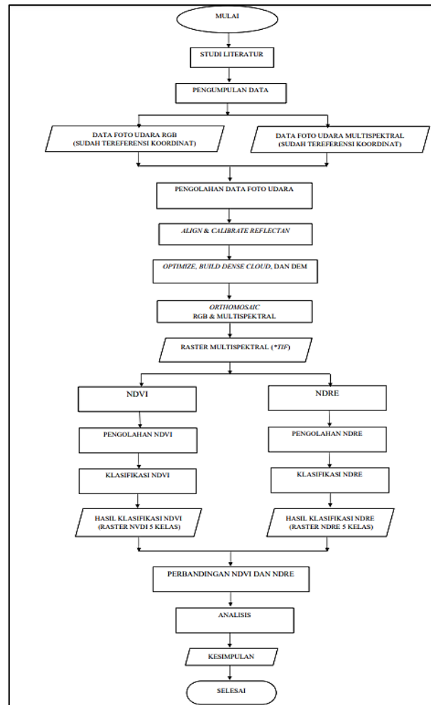
Gambar 2. Rancangan Penelitian
